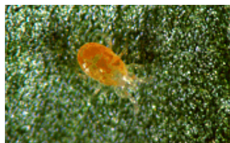
Amblyseius californicus
